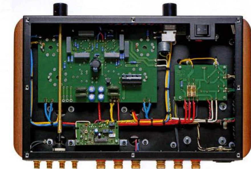
Sur cette vue de dessous, on note l'interrupteur de mise sous tension en haut à droite. La rigueur et la propreté du travail d'implantation sont exemplaires.
