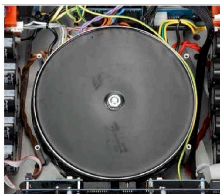
Transformateur d'alimentation de 2000 VA imprégné.
