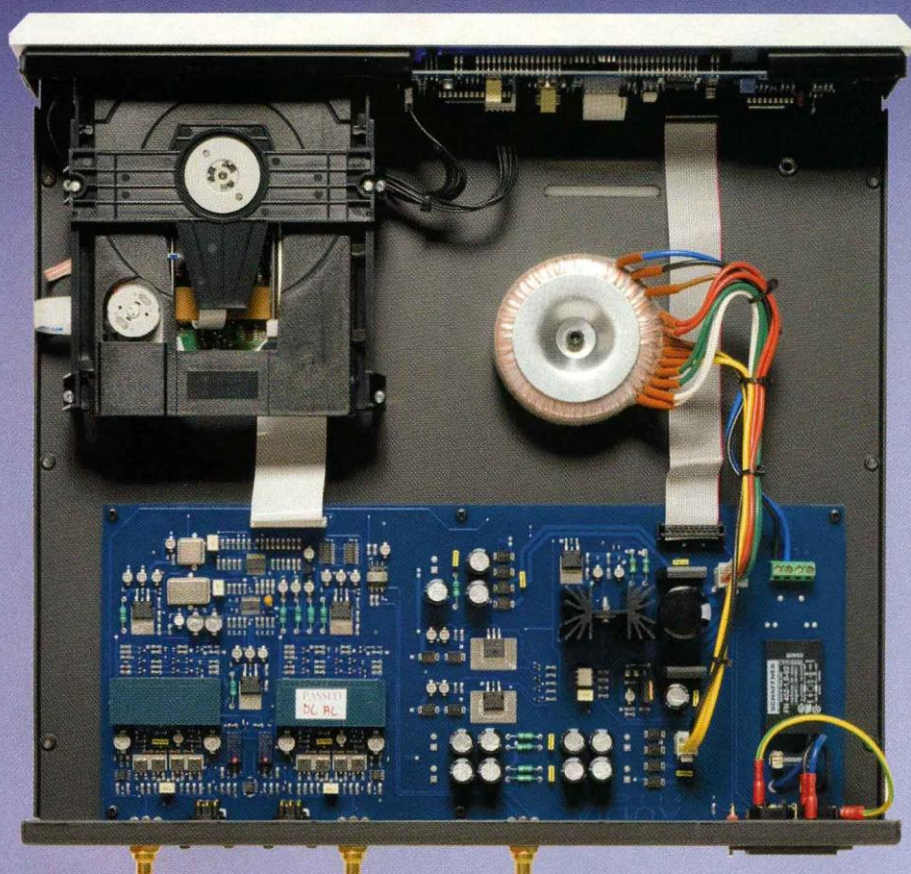
Difficile de faire plus ordonné que ce lecteur de CD italien. Toute l'électronique est regroupée sur un vaste circuit imprimé de grande qualité.
